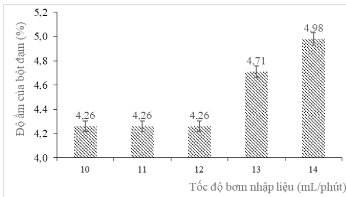
Hình 10. Ảnh hưởng của tốc độ bơm nhập liệu đến độ ẩm bột đậm sau sấy.
