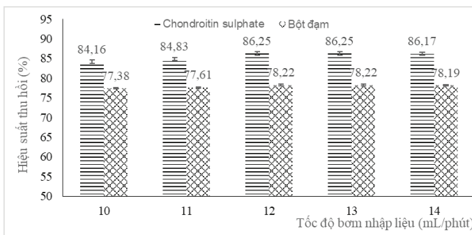
Hình 9. Ảnh hưởng của tốc độ bơm nhập liệu đến hiệu suất thu hồi chondroitin sulphate và bột đậm.
